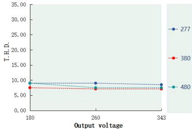
T.H.D. VS Output voltage(DL-240U-V343P-MUG)
