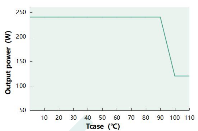
Output power VS Tcase (DL-240W-MXC)
