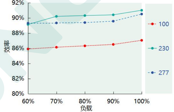
效率 VS. 负载 (DL-100Z-143A/P-MXL) (Io=0.7A)
