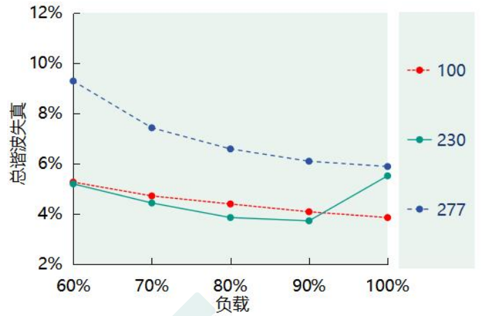
总谐波失真 VS.负载 (DL-100Z-56A/P-MXL)
