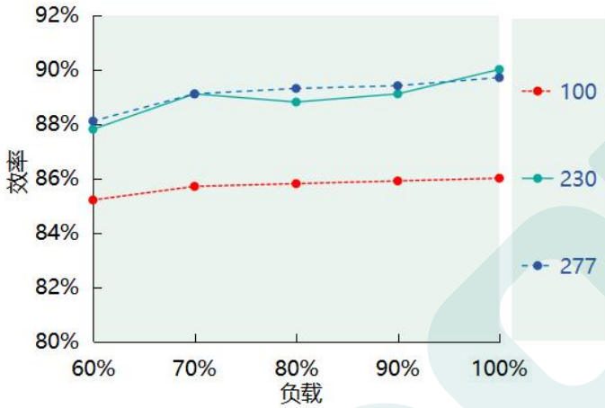
效率 VS. 负载 (DL-100Z-72A/P-MXL) (Io=1.39A)
