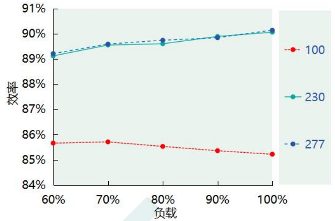
效率 VS. 负载 (DL-100Z-56A/P-MXL) (Io=1.79A)
