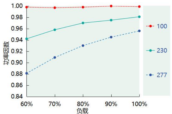
功率因素 VS. 负载 (DL-100Z-72A/P-MXL)
