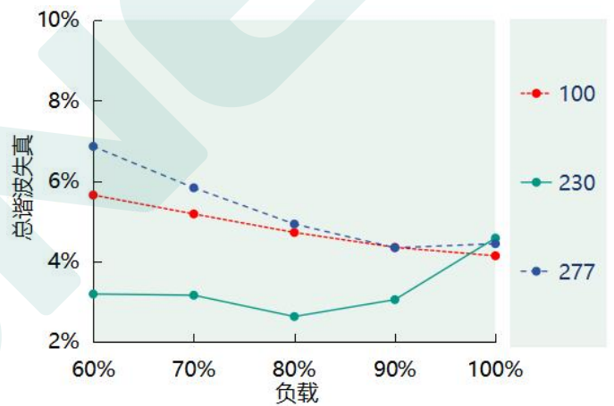
总谐波失真 VS.负载 (DL-100Z-143A/P-MXL)
