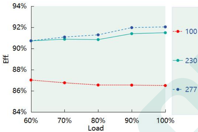
Eff. vs. Load ( DL-150Z-107A/P-MXL ) ( Io=1.4A )
