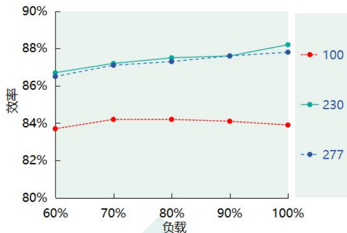
效率 VS. 负载 (Io=1.07A)
