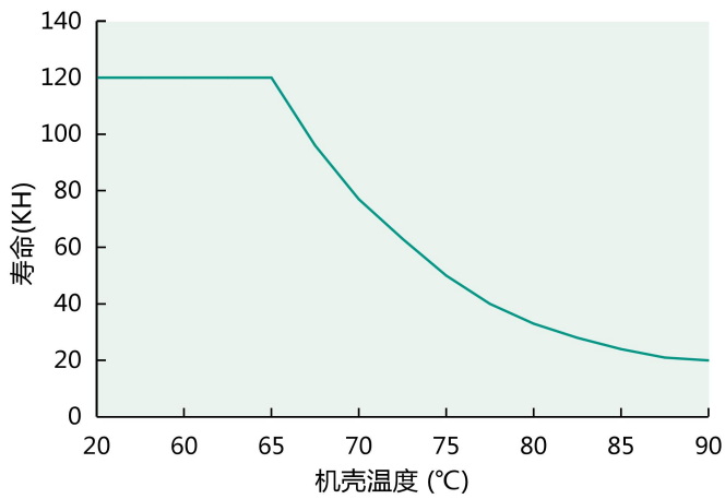
Tc VS 寿命(DL-80H-MXC)
