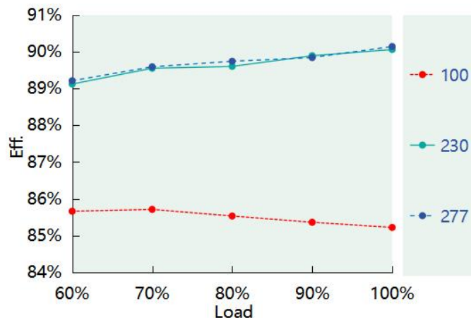
Eff. vs. Load( DL-100Z-56A/P-MXL )( Io=1.79A )
