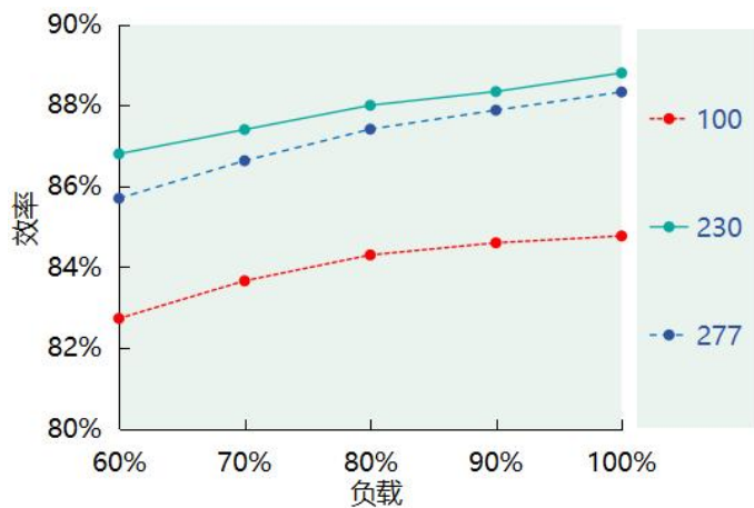
效率 VS. 负载 (DL-50Z-72A/P-MXL) ( I_o=0.7A )
