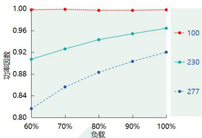
功率因素 VS. 负载 (DL-50Z-72A/P-MXL)
