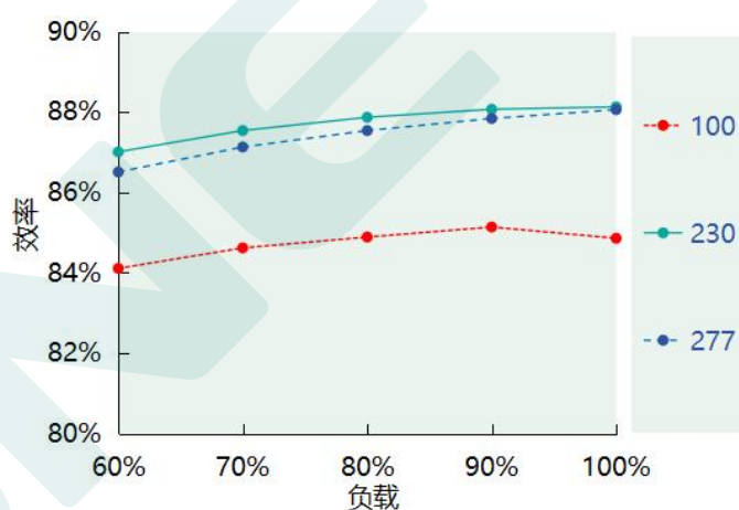
效率 VS. 负载 (DL-50Z-56A/P-MXL) (Io=0.9A)
