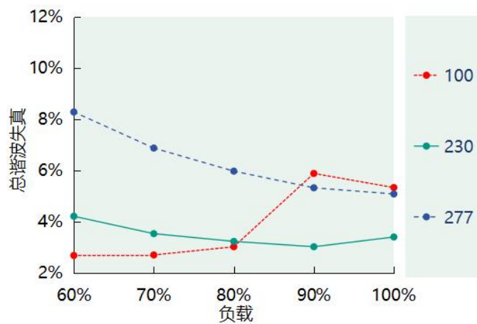
总谐波失真 VS. 负载 (DL-50Z-56A/P-MXL)
