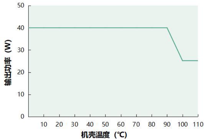
输出功率 VS 机壳温度(DL-40H-MXC)
