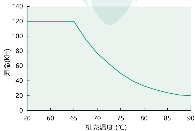
Tc VS 寿命(DL-40H-MXC)
