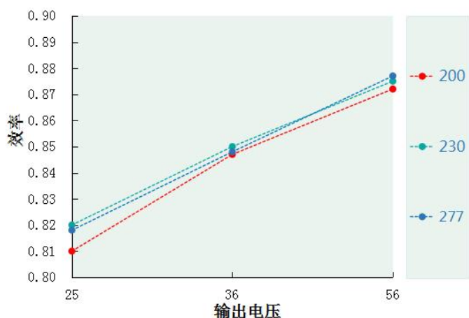
效率 VS 输出电压 DL-40H-56A/P-MXC
