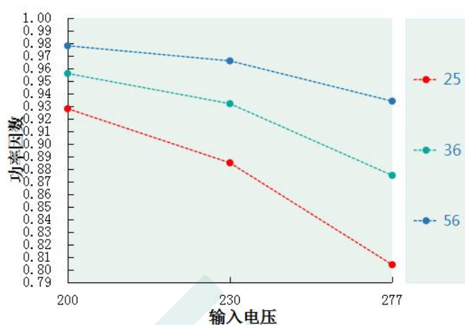
功率因素 VS 输入电压 DL-40H-56A/P-MXC
