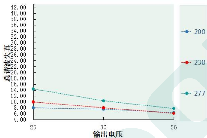
总谐波失真 VS 输出电压 DL-40H-56A/P-MXC
