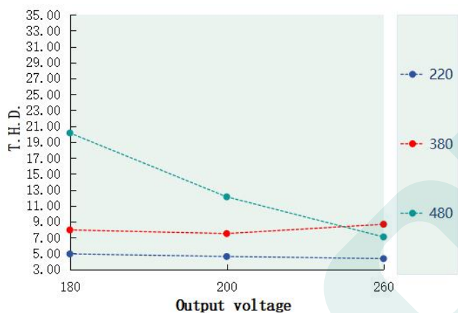
T.H.D. VS Output voltage ( DL-200V-260A/S/X-PXG )
