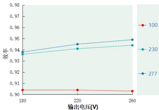
效率 VS 输出电压 DL-80Z-260A/S/X-PXG
