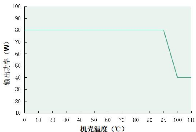
输出功率 VS 机壳温度(DL-80Z-260A/S/X-PXG)
