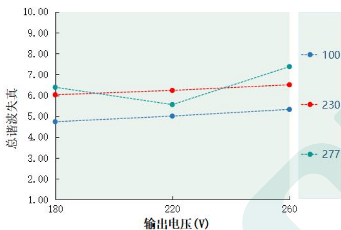
总谐波失真 VS 输出电压 DL-80Z-260A/S/X-PXG
