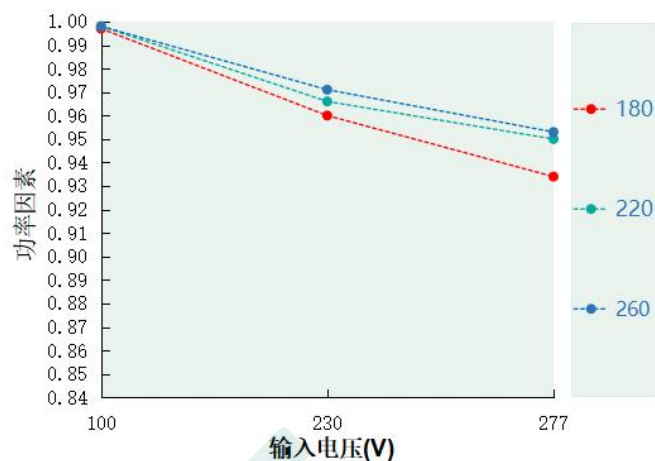
功率因素 VS 输入电压 DL-80Z-260A/S/X-PXG
