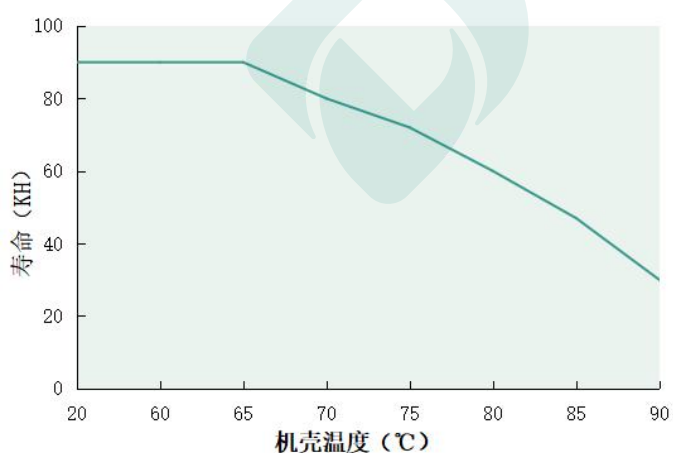
寿命 VS 机壳温度(DL-80Z-260A/S/X-PXG)
