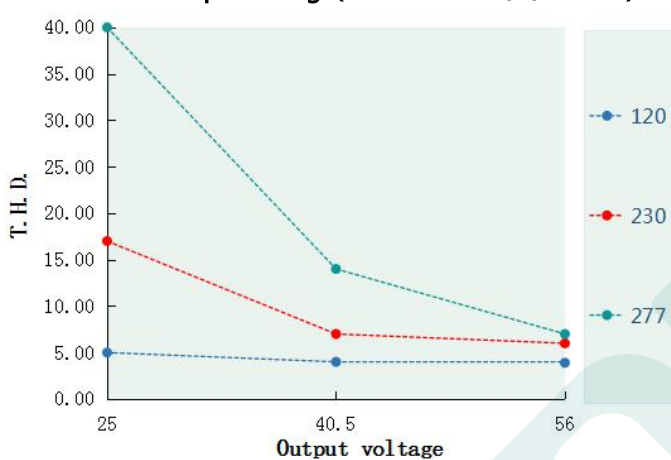
T.H.D. VS Output voltage(DL-75W-V56A/P/X-MDK)
