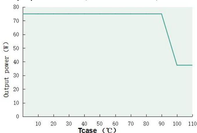
Output power VS Tcase (DL-75W-A/P/X-MDK)
