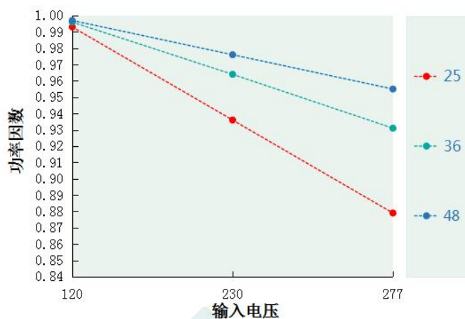
功率因素 VS 输入电压 DL-50W-V48S/X-MTG
