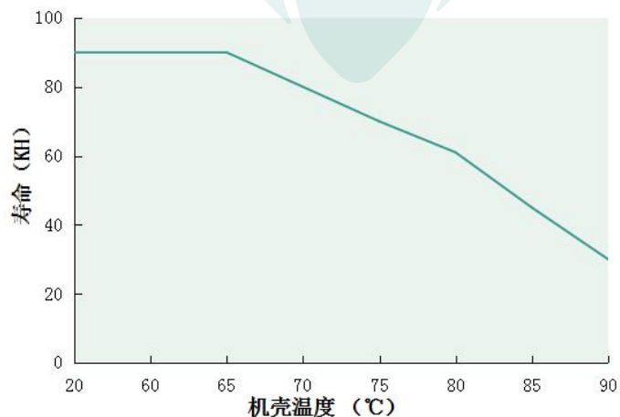
Tc VS 寿命 DL-50W-S/X-MTG
