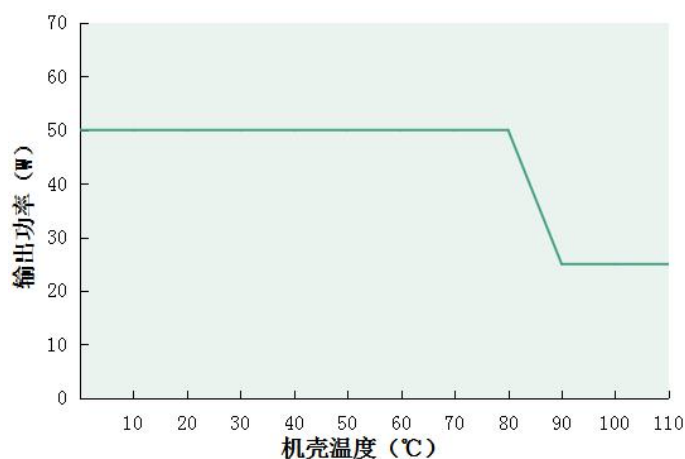
输出功率 VS 机壳温度 DL-50W-S/X-MTG
