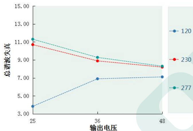
总谐波失真 VS 输出电压 DL-50W-V48S/X-MTG
