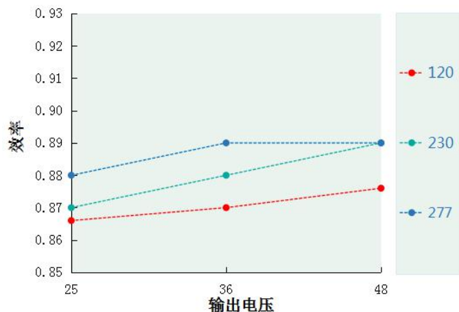
效率 VS 输出电压 DL-50W-V48S/X-MTG
