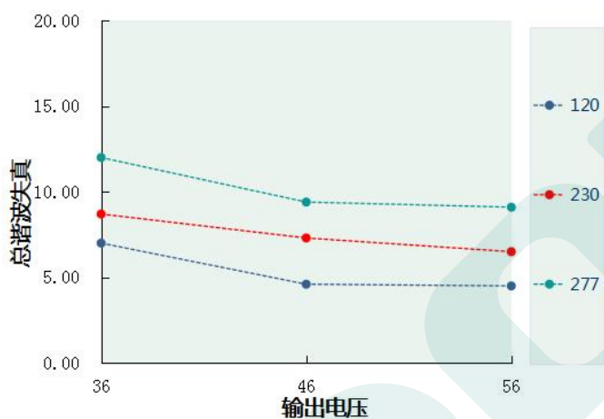
总谐波失真 VS 输出电压 DL-1000Z-56X/J-MXS
