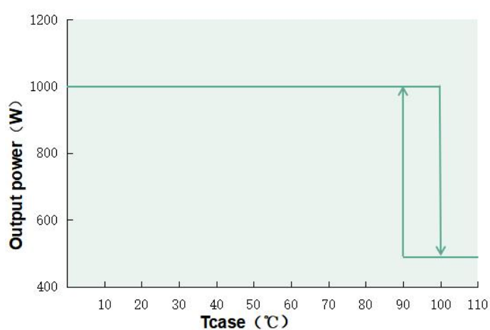
输出功率 VS 机壳温度 (DL-1000Z-56X/J-MXS)
