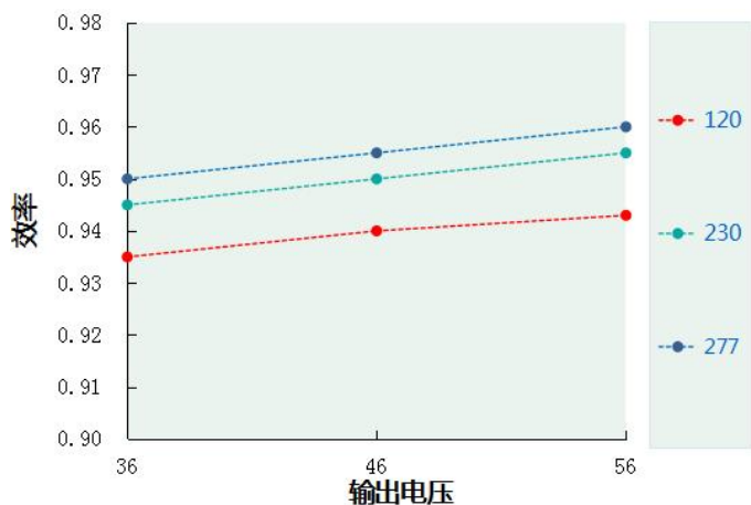
效率 VS 输出电压 DL-1000Z-56X/J-MXS
