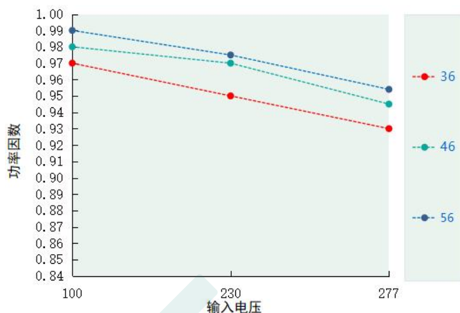
功率因素 VS 输入电压 DL-1000Z-56X/J-MXS
