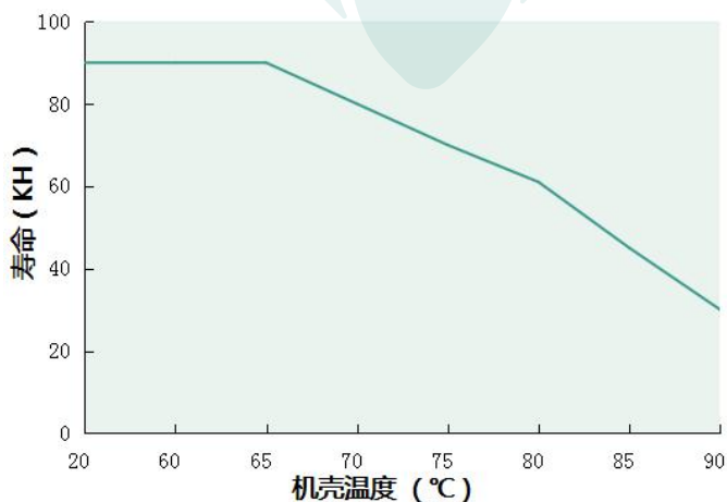
Tc VS 寿命 (DL-1000Z-56X/J-MXS)
