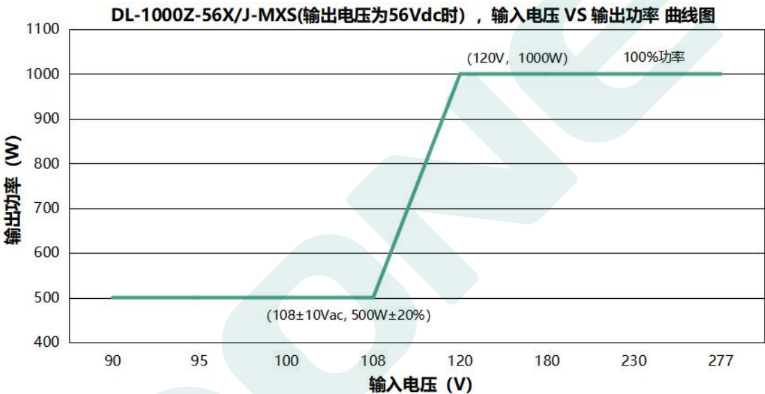
DL-1000Z-56X/J-MXS(输出电压为 56Vdc 时，不同输入电压对应的额定输出电流值和输出功率)
