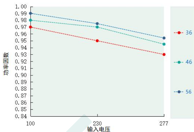
功率因素 VS 输入电压 DL-1200Z-56X-MXS
