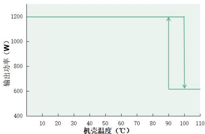
输出功率 VS 机壳温度 (DL-1200Z-56X-MXS)
