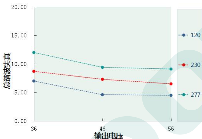
总谐波失真 VS 输出电压 DL-1200Z-56X-MXS
