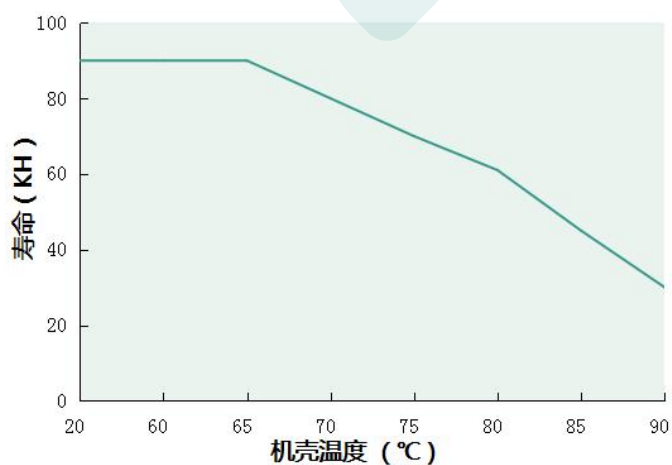
Tc VS 寿命 (DL-1200Z-56X-MXS)
