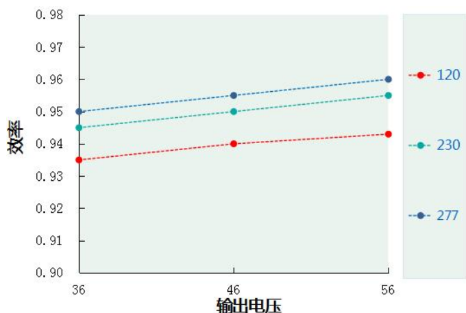
效率 VS 输出电压 DL-1200Z-56X-MXS
