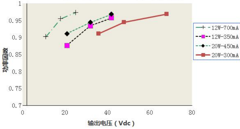
■ 输出电压 VS 功率因素
