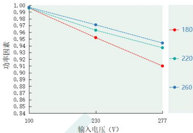
功率因素 VS 输入电压 DL-200Z-260X-PXS
