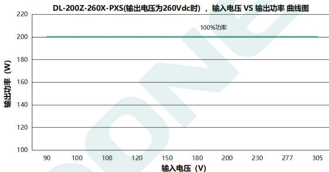
DL-200Z-260X-PXS(输出电压为 260Vdc 时，不同输入电压对应的额定输出电流值和输出功率)
