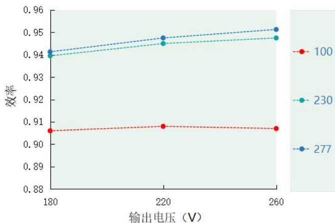
效率 VS 输出电压 DL-200Z-260X-PXS
