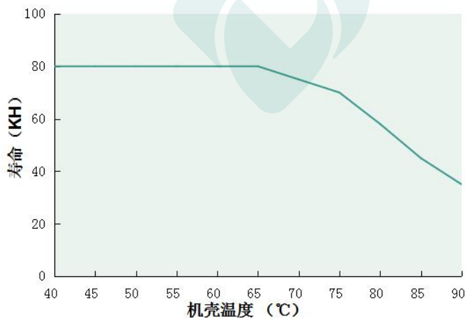
机壳温度 VS 寿命 DL-200Z-260X-PXS
