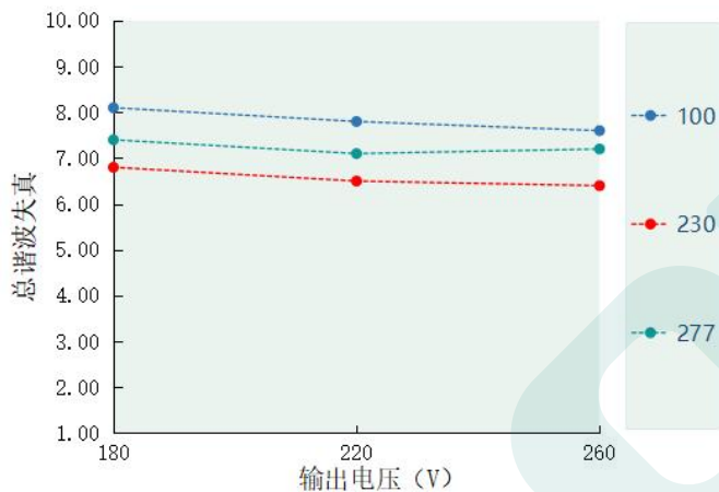
总谐波失真 VS 输出功率 DL-200Z-260X-PXS
