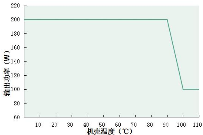
输出功率 VS 机壳温度 DL-200Z-260X-PXS
