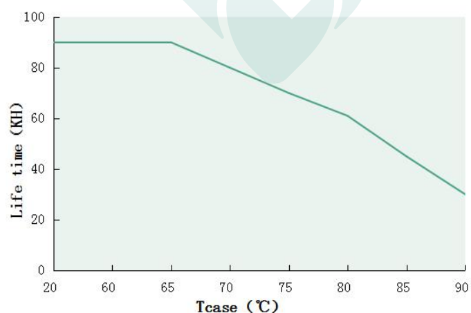
Tcase VS Lifetime(DL-150W-A/P/X-MDK)
