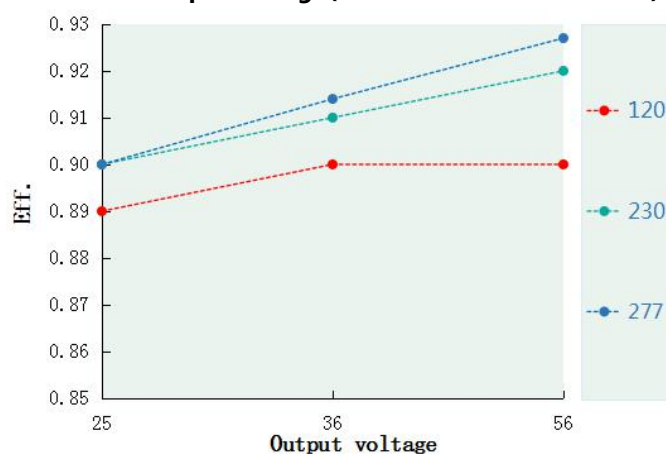
Eff. VS Output voltage(DL-150W-V56A/P/X-MDK)
