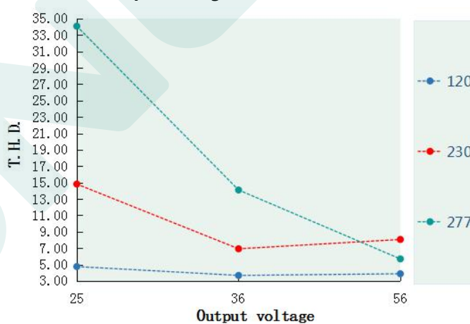
T.H.D. VS Output voltage(DL-150W-V56A/P/X-MDK)
