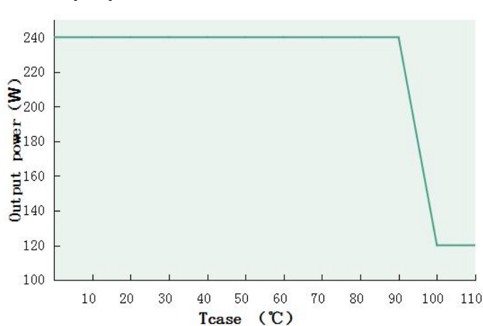
Output power VS Tcase (DL-150W-A/P/X-MDK)
