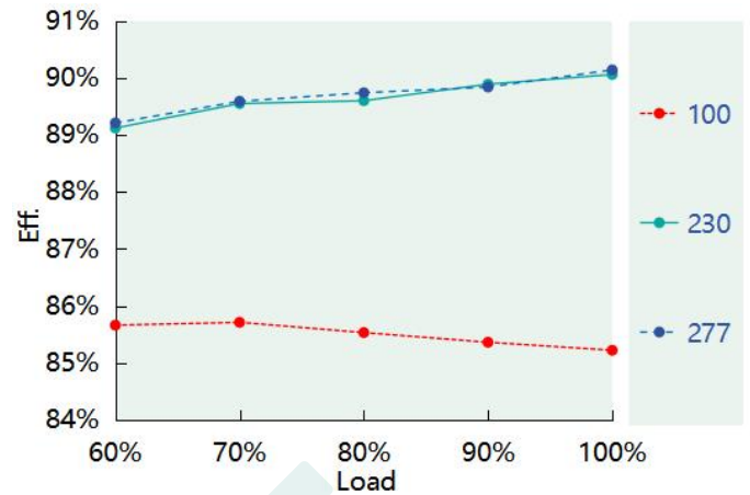
Eff. vs. Load (DL-100Z-56A/P-MXL)
