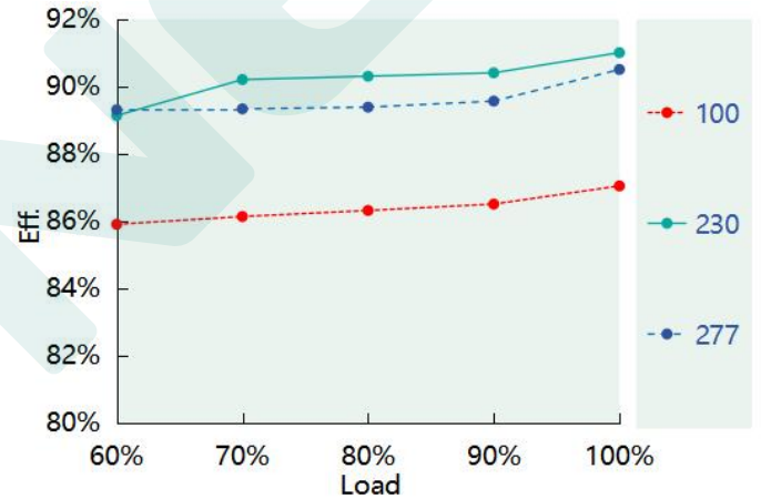
Eff. vs. Load (DL-100Z-143A/P-MXL)
