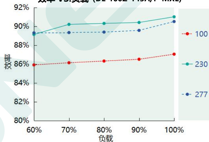
效率 VS. 负载 (DL-100Z-143A/P-MXL)
