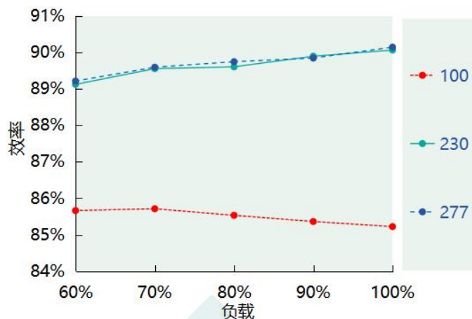
效率 VS. 负载 (DL-100Z-56A/P-MXL)
