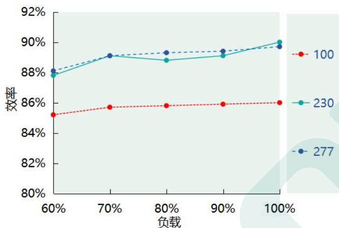
效率 VS. 负载 (DL-100Z-72A/P-MXL)
